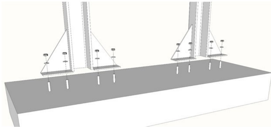
Montera skyltstativ på fundament enligt principalskiss ovan
