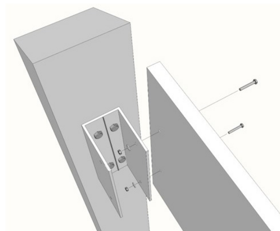
Skytarna monteras på cortenbeslag enligt bild
